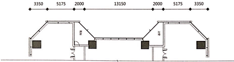
九、十一、十三、十五、十七层局部平面图
